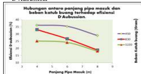
Gambar 6 Grafik hubungan antara panjang pipa masuk dan beban katub buang terhadap efisiensi D'Aubussion
