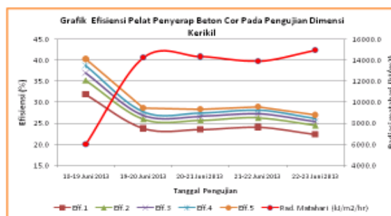
Gambar 7 Grafik Efisiensi Pelat Penyerap Beton Cor
