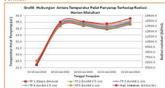
Gambar 5. Grafik Hubungan Temperatur Kaca Terhadap Radiasi Harian Matahari
