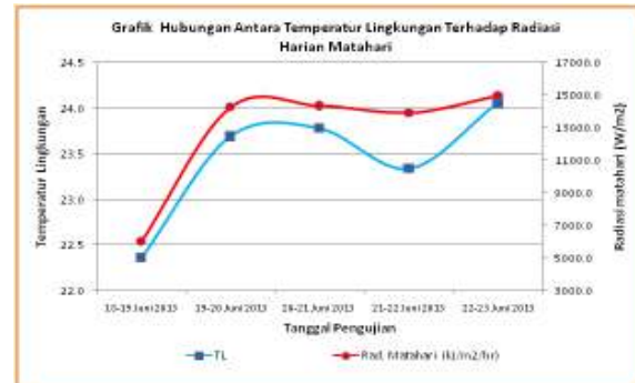
Gambar 4. Hubungan temperatur lingkungan terhadap radiasi harian matahari.
