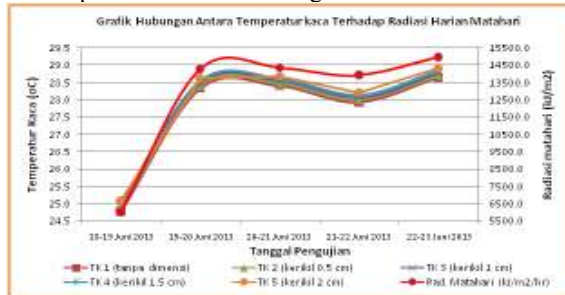
Gambar 6 Grafik Hubungan Temperatur Kaca Terhadap Radiasi Harian Matahari
