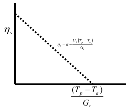
Gambar 1. Grafik karakteristik efisiensi penyerapan pelat penyerap (Sumber: Duffie dan Beckman. 1980:251)
