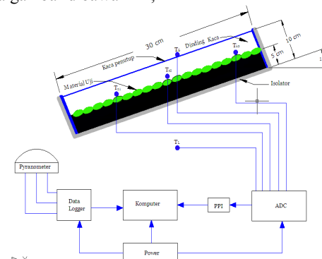
Gambar 3. Skema uji penyerap panas radiasi matahari
