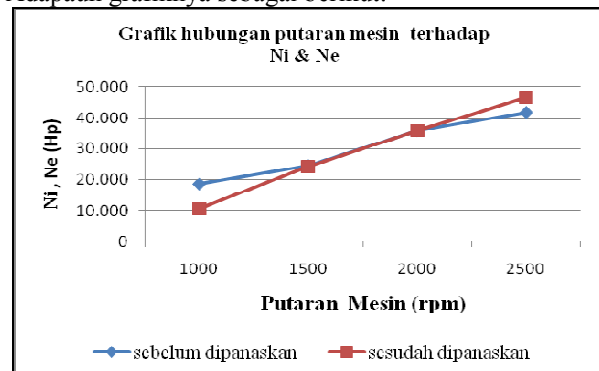
Gambar 9. Grafik hubungan putaran mesin dengan daya indikasi (Ni) dan daya efektif (Ne)
