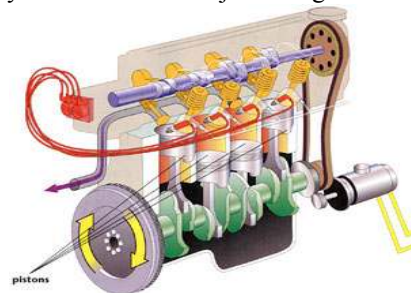
Gambar 3 Proses pembakaran ( www.ringdiesel-bensin.com )
