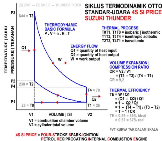
Gambar 4. siklus thermodinamika Otto
