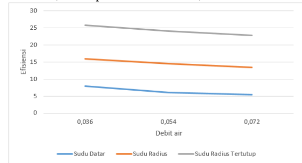
Gambar 6 Grafik beda sudu terhadap efisiensi
