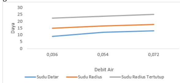
Gambar 5 Grafik beda sudu terhadap daya
